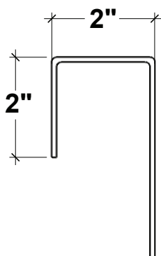
ROUNDED EDGE TRIM
