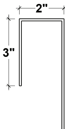
STANDARD SQUARE EDGE TRIM
